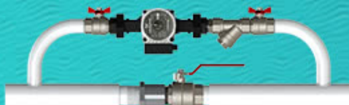
Байпасный узел в сборе
